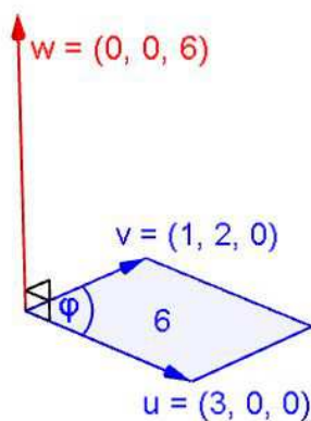
Obrázek 39: |\vec{w}| = |\vec{u}||\vec{v}| \sin \varphi
