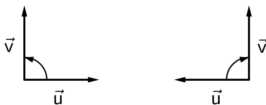
Obrázek 36: Pravotočivá (vlevo) a levotočivá (vpravo) báze prostoru V_2
