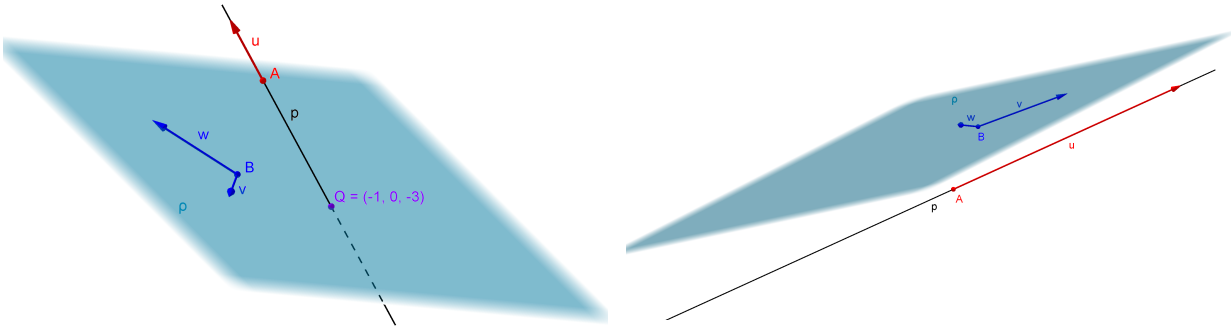
a) p, \rho jsou různoběžné
