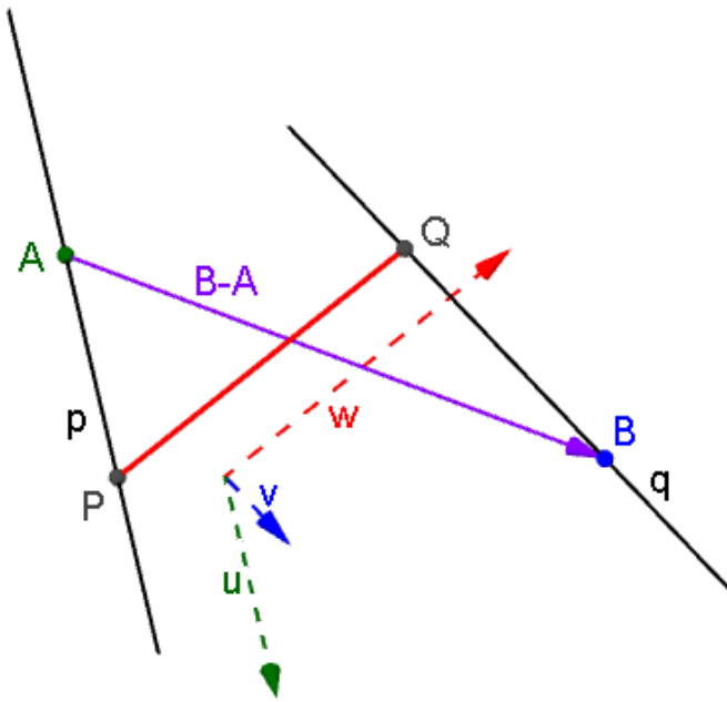
Obrázek 70: Vzdálenost dvou mimoběžek p, q je rovna délce jejich nejkratší příčky PQ , která je kolmá k oběma přímkám.
