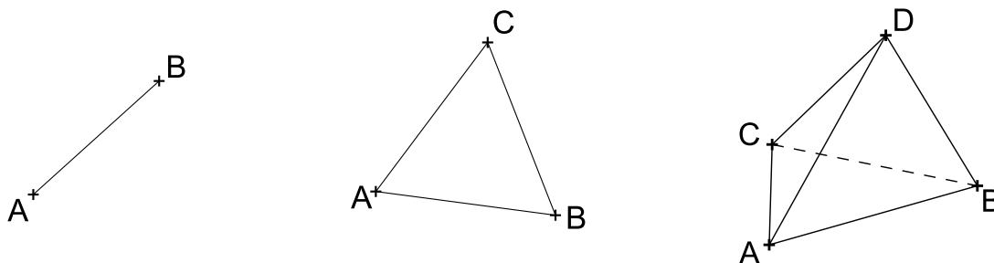
Obrázek 50: Úsečka, trojúhelník a čtyřstěn jako simplex v bodových prostorech 1, 2 a 3, v daném pořadí
