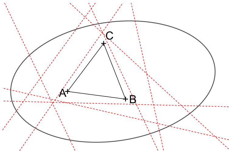
Obrázek 49: Konvexním obalem 3 lineárně nezávislých bodů A, B, C je trojúhelník \triangle ABC
