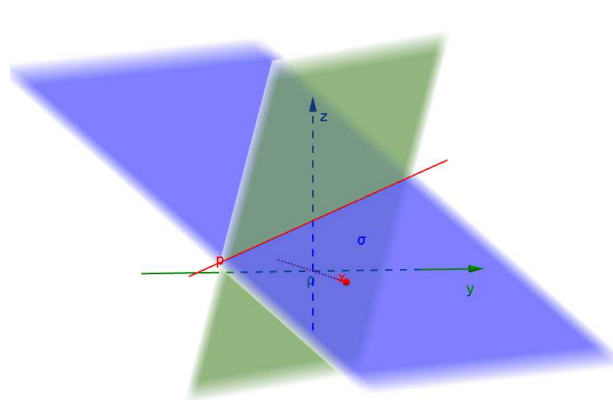
a) Svazek rovin 1. druhu
