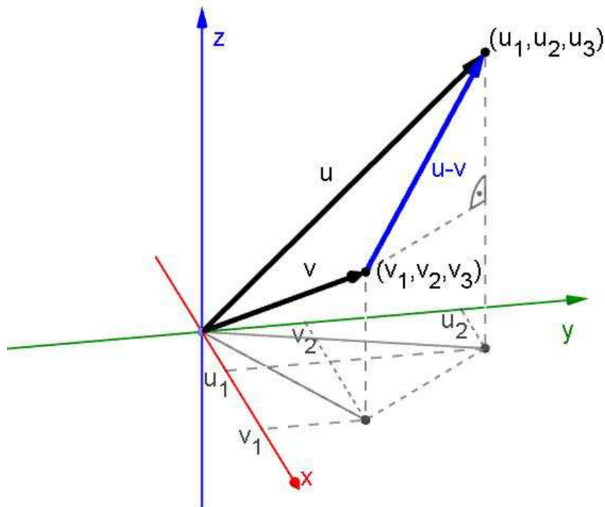
Obrázek 15: Vztah pro velikost vektoru \vec{u} - \vec{v} obsahuje formuli pro výpočet Eukleidovského skalárního součinu
